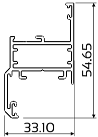
DIE No. W57602 Cas 30.5 Sash Euro
