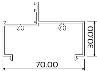
DIE No. W70968 Frame 70mm
