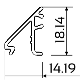
DIE No. W35620 Cas30.5 Bead Euro 13mm Gap
