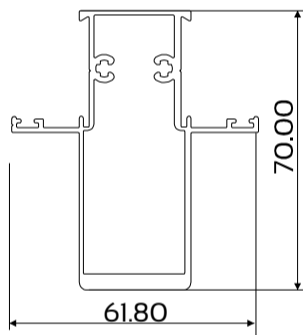
DIE No. W54652A Cas30.5 Mullion 70mm
