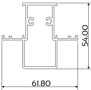
DIE No. W54651A Cas30.5 Mullion 54mm
